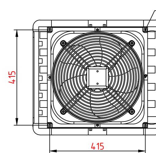
Вид сзади
