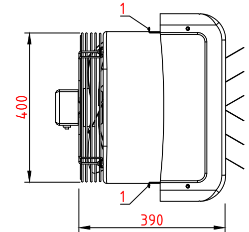
Вид сбоку
